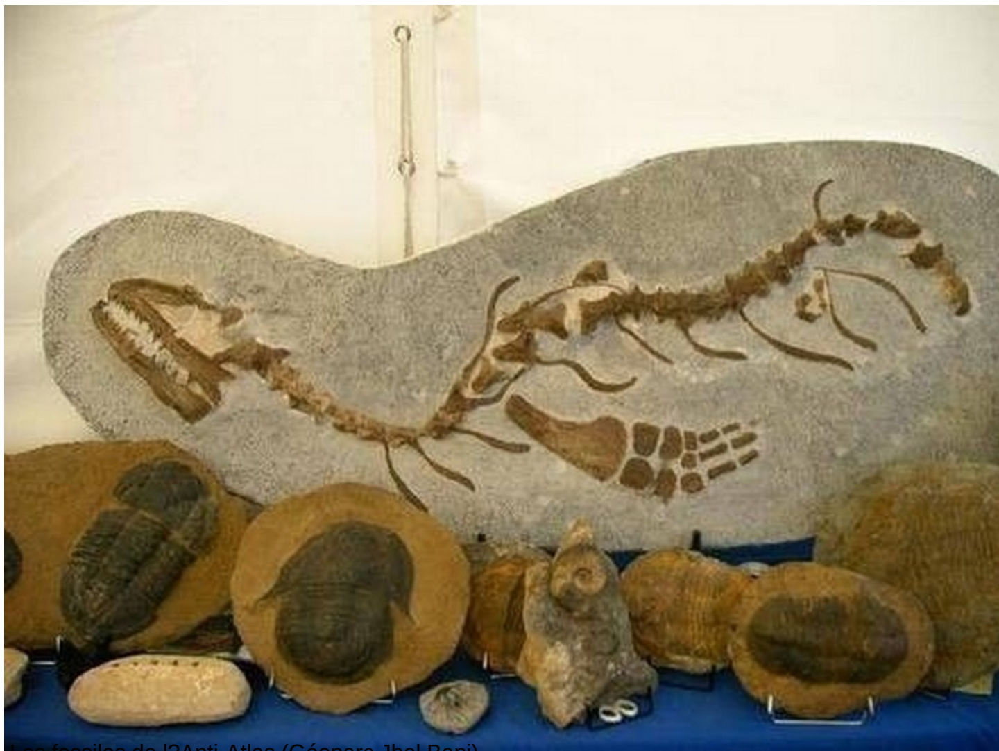
Les fossiles de l'Anti-Atlas (Géoparc Jbel Bani)
